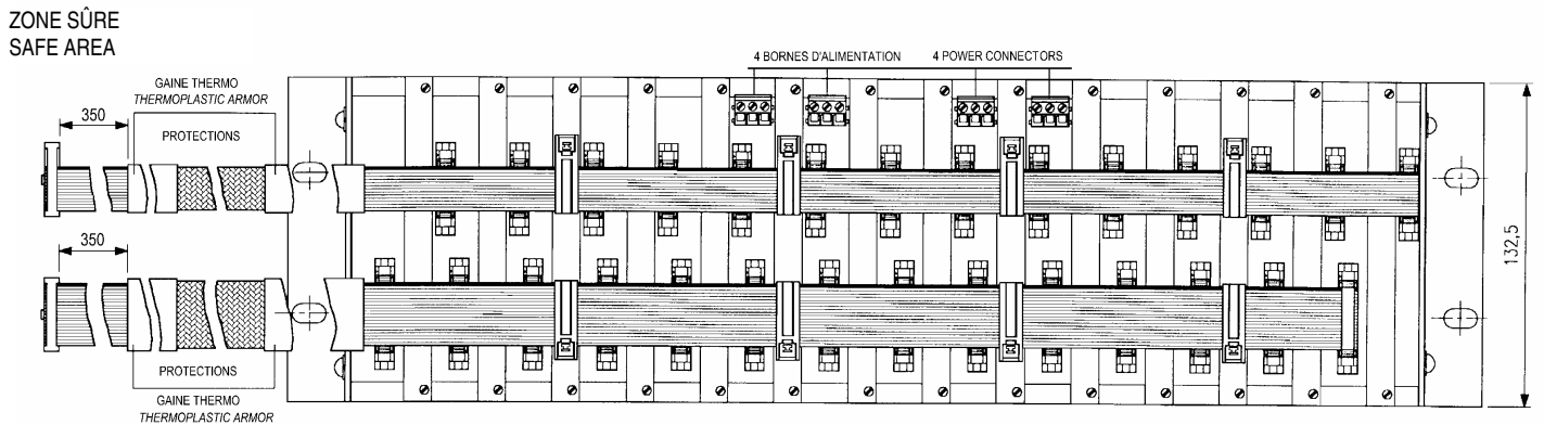
VUE ARRIERE PA 1154 (châssis pivotant) / BACK VIEW PA 1154 (rotating frame)
